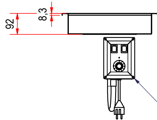
Betjeningspanel : utsparingsmål 107mm x 155mm
